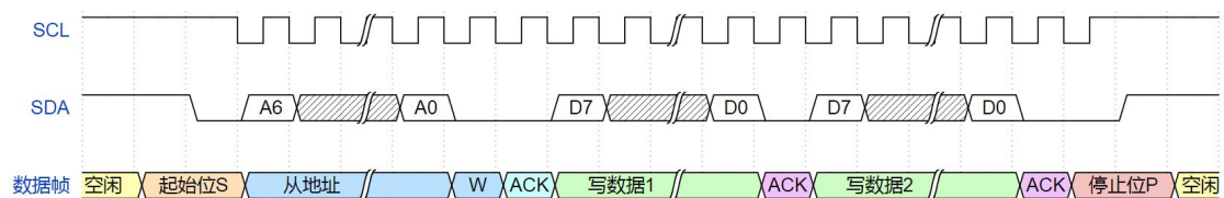
图 7：连续写数据操作时序图
