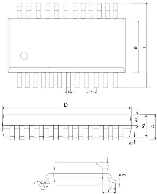
图 10：封装尺寸图
