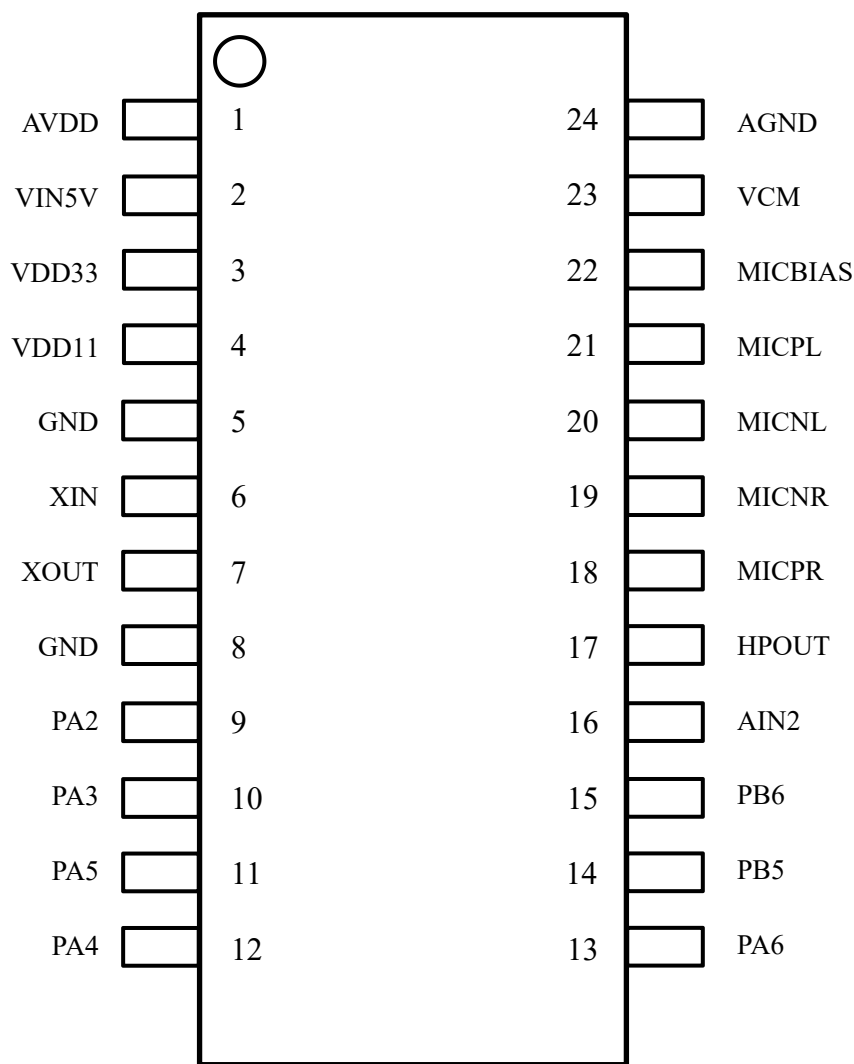
图 2： SSOP24 引脚图
