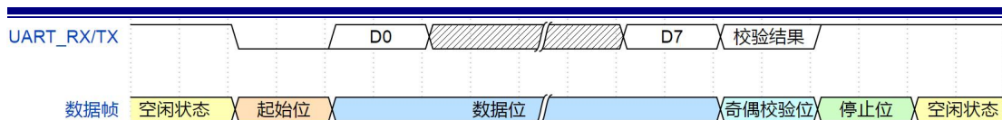
图 3：数据帧时序图 1
